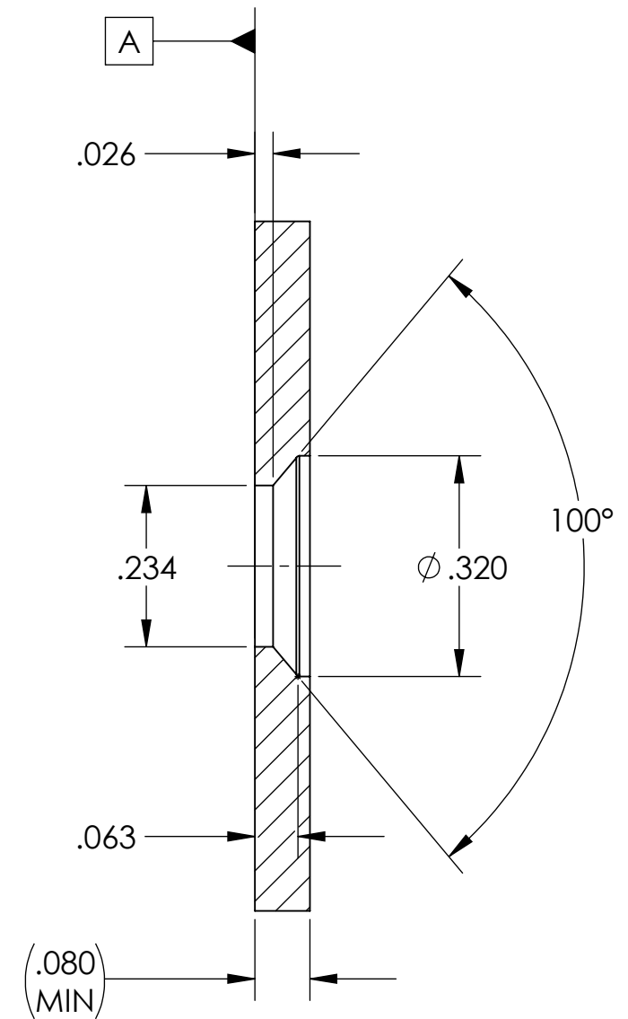
SECTION A-A SCALE 4 : 1
